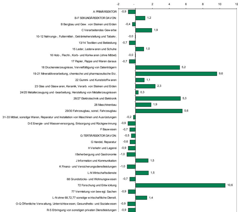
Abbildung 43: Förderungslokationskoeffizienten 35 SFG 2009
