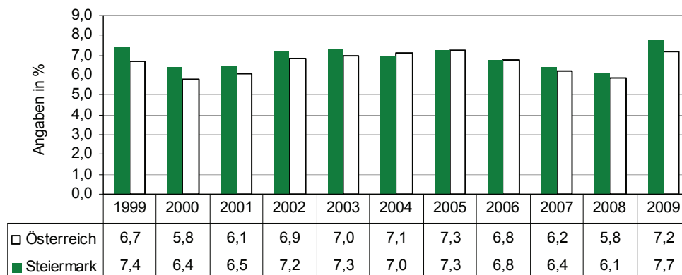
Abbildung 22: Arbeitslosenquoten 1999-2009
